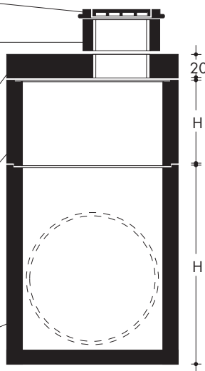
SEZIONE
