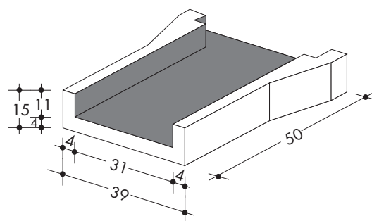
ASSONOMETRIA
