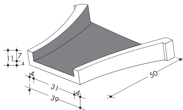
ASSONOMETRIA
