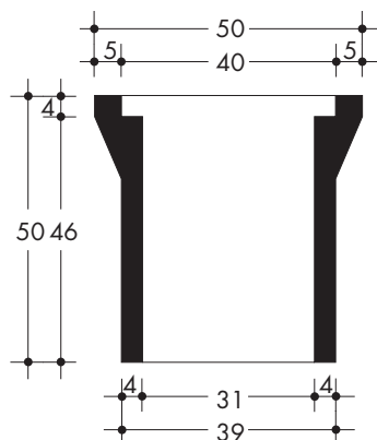
PIANTA
