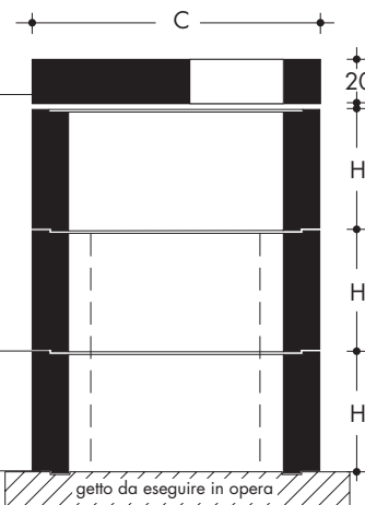
SEZIONE
